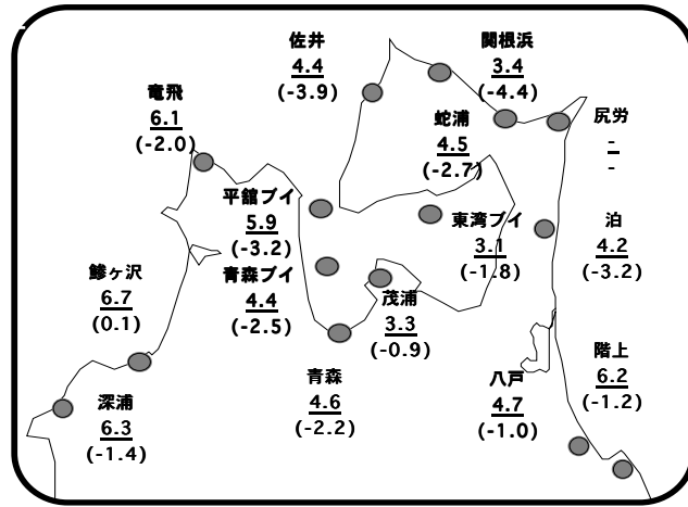
図 定地水温 (2月1～5日) 平均値 (平年差) ブイ1m
