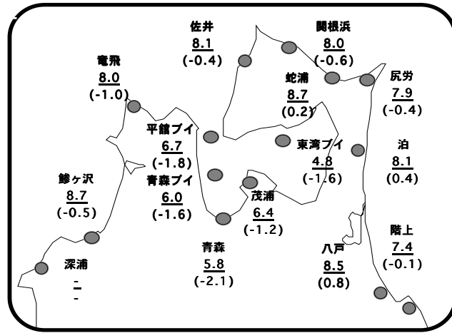
図 定地水温 (4月11～15日) 平均值 (平年差) ブイ1m
