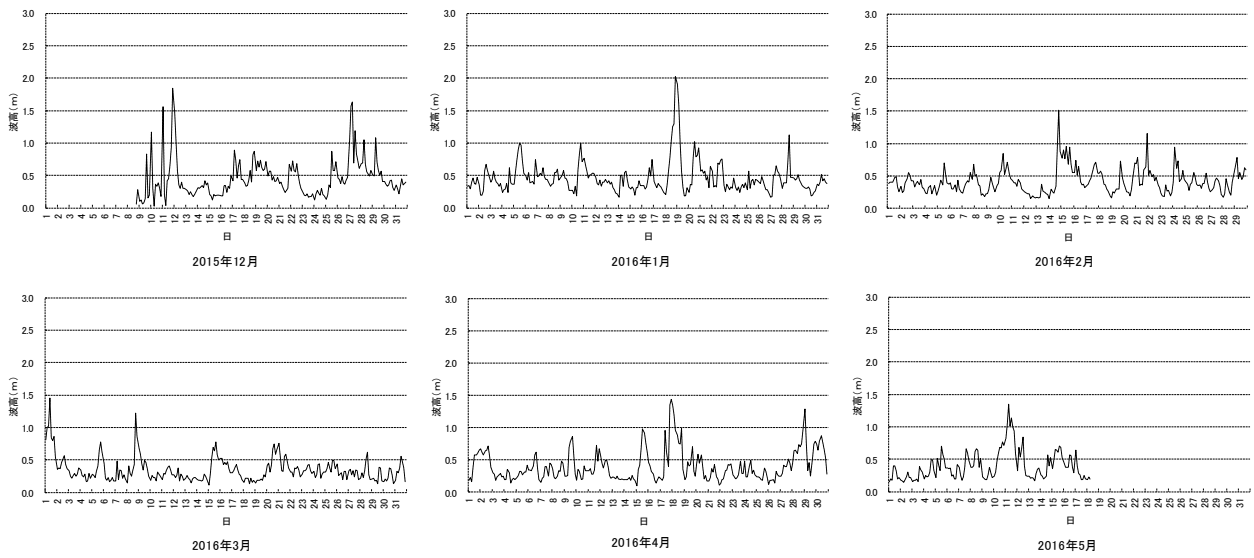
図 4. 後潟沖における有義波高
