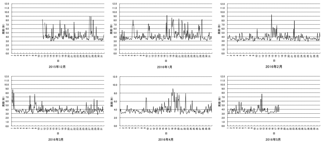
図 5. 後潟沖における有義周期
