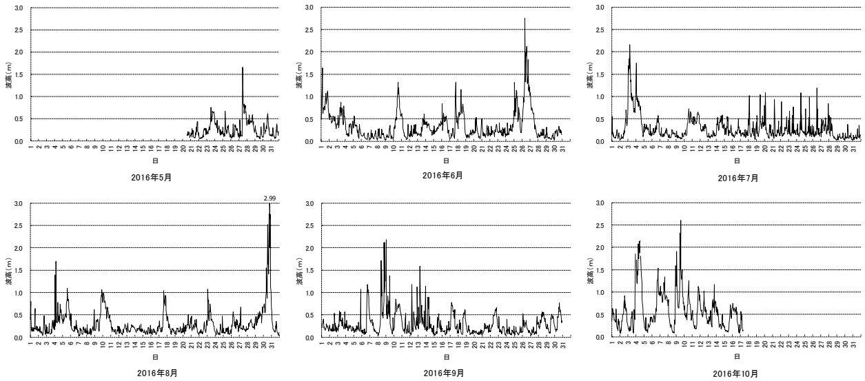
図 6. 浜奥内沖における有義波高
