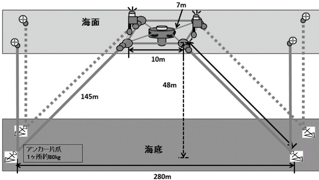
図 3. 設置方法（4点係留）
