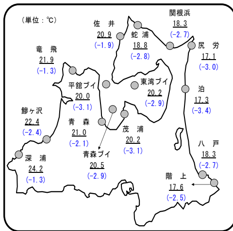
図 定地水温(8月16日～20日) 平均値(平年差)ブイは1m
