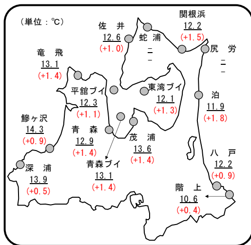
図 定地水温(5月16日～20日) 平均値(平年差)ブイは1m
