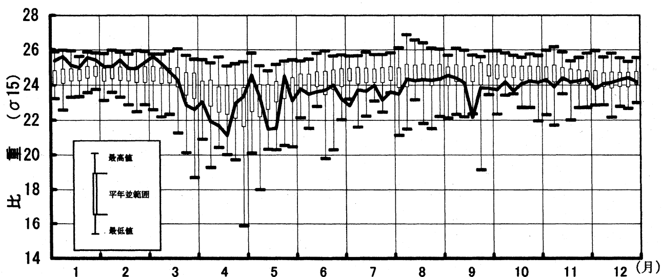
図3 茂浦における半月平均比重の推移 (2000年) (箱ヒゲの統計期間1968～2000年)
