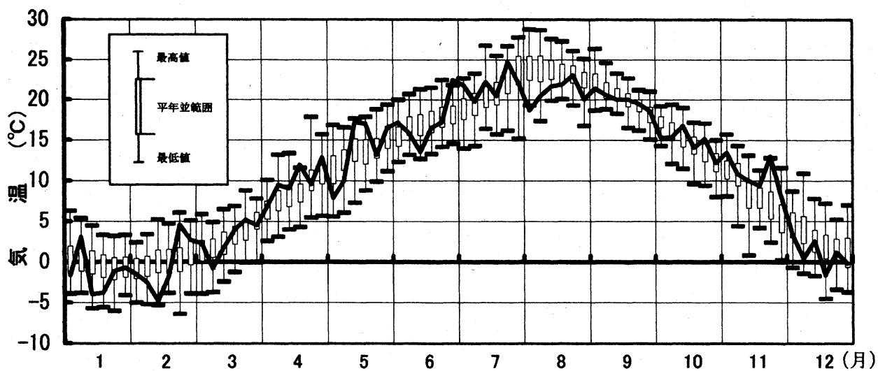
図1 茂浦における半月平均気温の推移 (2001年) (箱ヒゲの統計期間1968～2000年)
