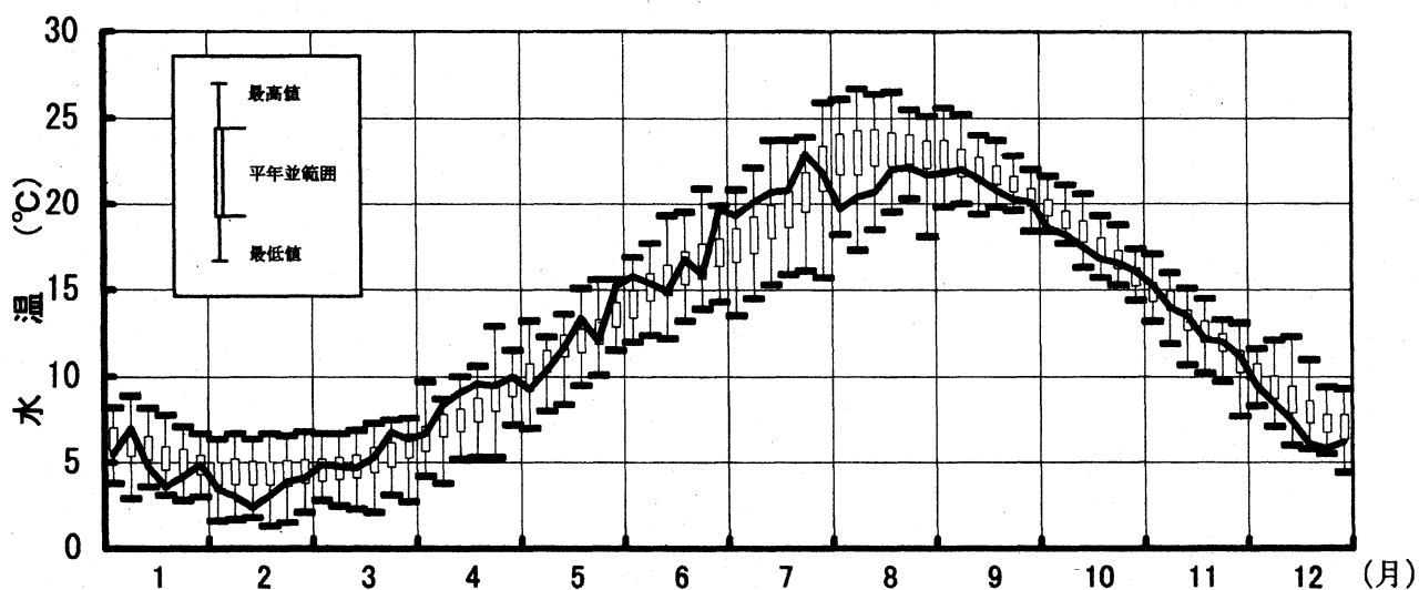
図2 茂浦における半月平均水温の推移 (2000年) (箱ヒゲの統計期間1968～2000年)
