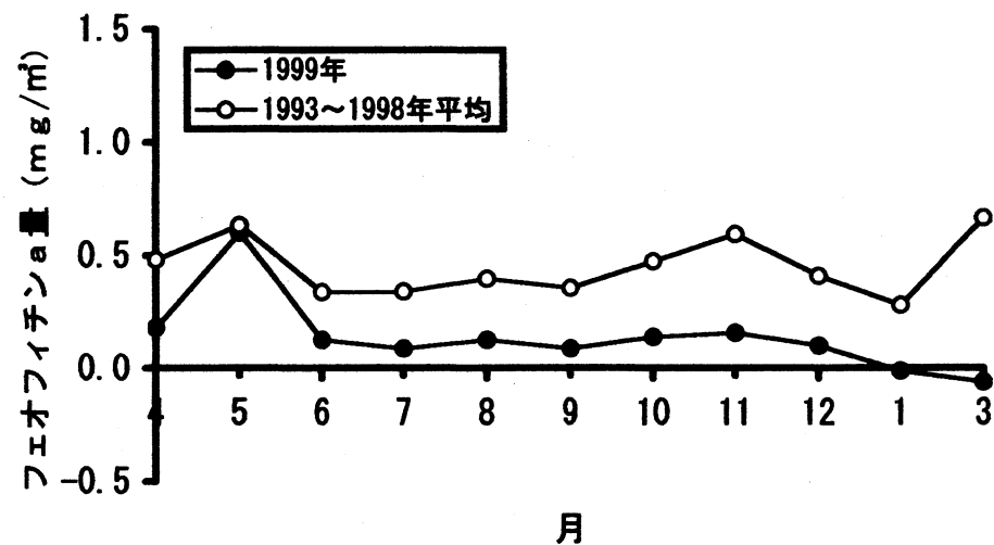
図4 西湾湾央部におけるフェオフィチンa量の推移
