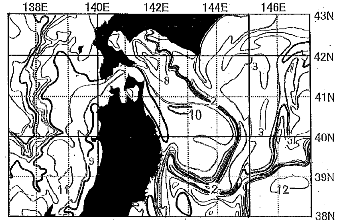
資料：(社)漁業情報サービスセンター 北部太平洋海況速報 第83号 1月20日発行
