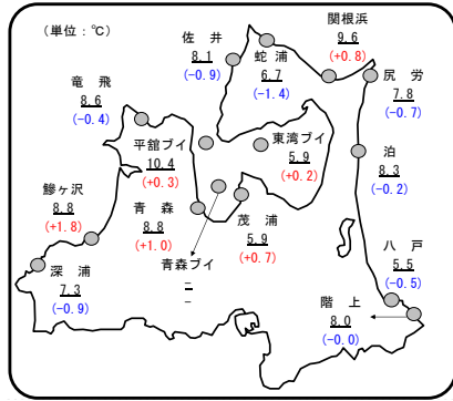
図 定地水温(1月16～20日) 平均值(平年差)1m
