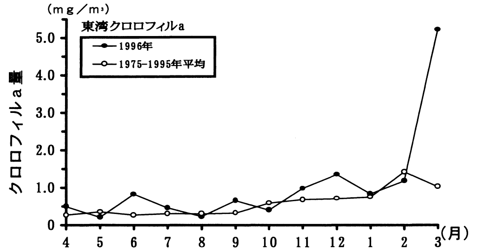
図4 東湾湾中央部におけるクロロフィル a の分布状況 (1996年 : 0、20、40m層平均)
