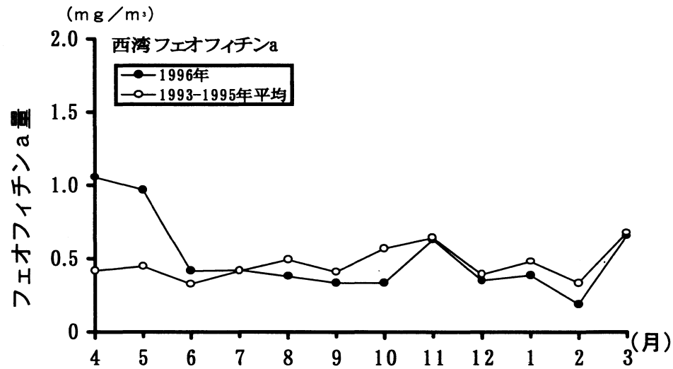
図3 西湾湾中央部におけるフェオフィチン a の分布状況 (1996年 : 0、20、40m層平均)
