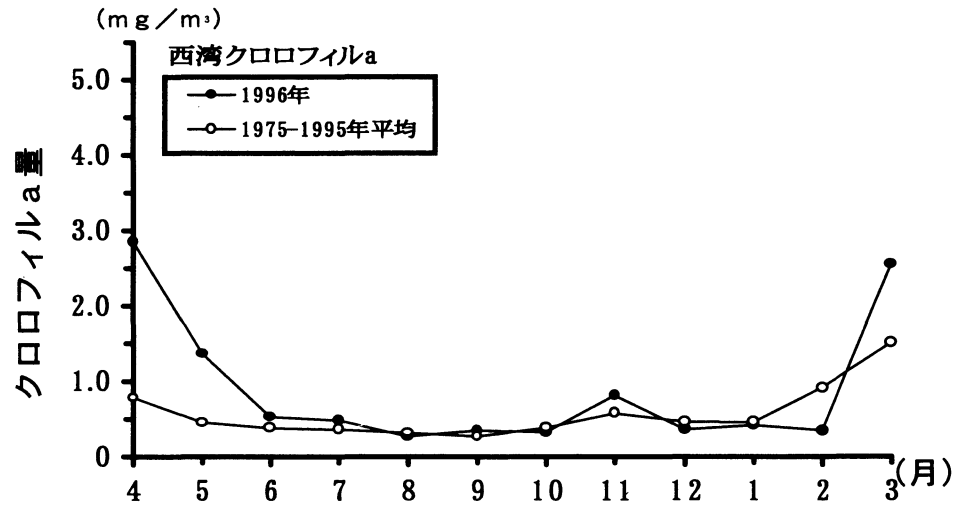
図5 東湾湾中央部におけるフェオフィチン a の分布状況 (1996年 : 0、20、40m層平均)
