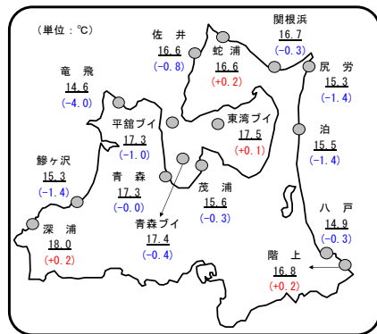
図 定地水温(10月26～31日) 平均値(平年差) 1m
