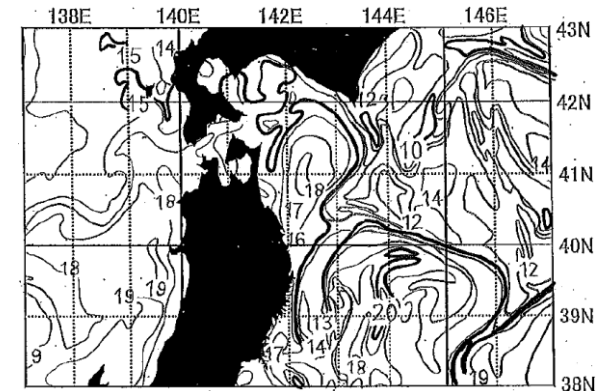
資料：(社)漁業情報サービスセンター 北部太平洋海況速報 第63号 11月4日発行
