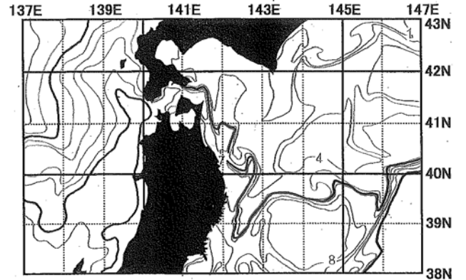
資料: (社) 漁業情報サービスセンター 北部太平洋海況速報 第85号 1月31日発行 (表面水温分布)
