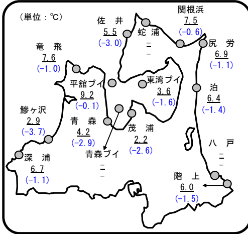
図 定地水温(1月26~31日) 平均値(前年差)ブイ1m
