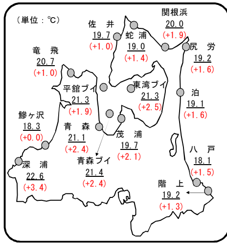
図 定地水温(10月16～20日) 平均値(前年差)ブイ1m
