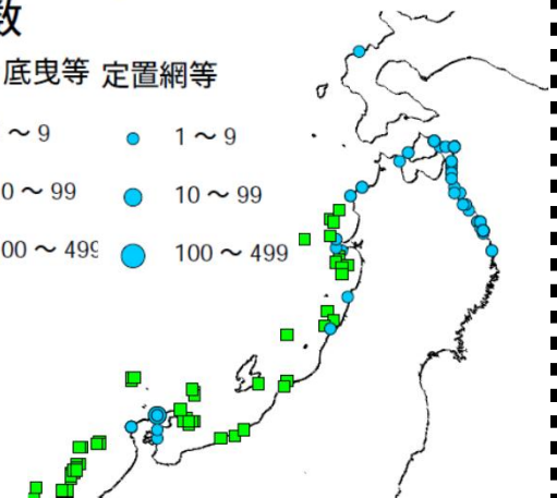
資料：(社) 漁業情報サービスセンター 北部太平洋海況速報 第58号 10月19日発行
