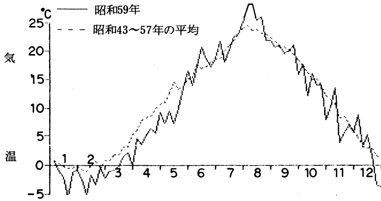
第1図 気温（半旬平均値）とその平年偏差の推移
