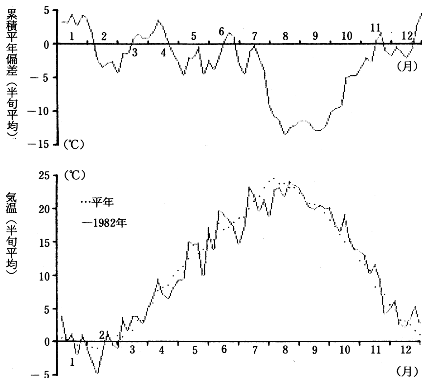
図-1 気 温 (1982年)
