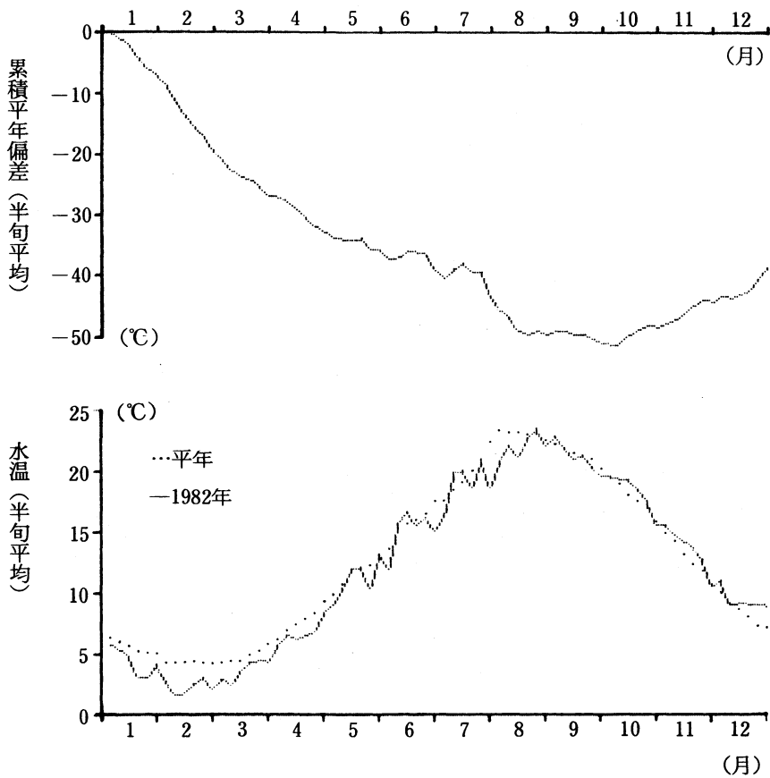
図-2 水 温 (1982年)
