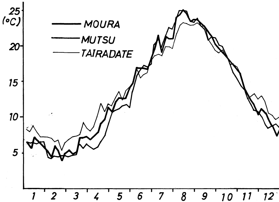
第1図 昭和47年表層水温半月平均
