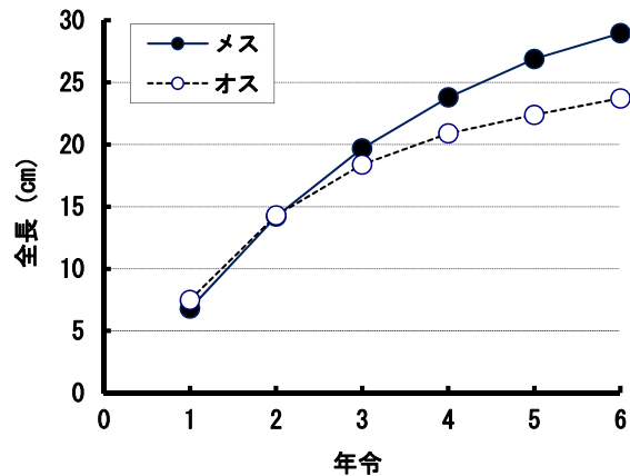
図 青森県におけるマガレイの成長
