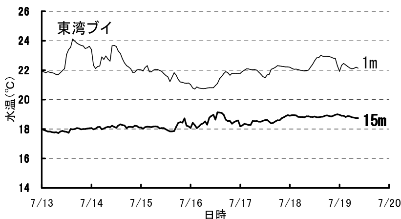
図1 各ブイでの1mおよび15m層の毎時の水温変化
