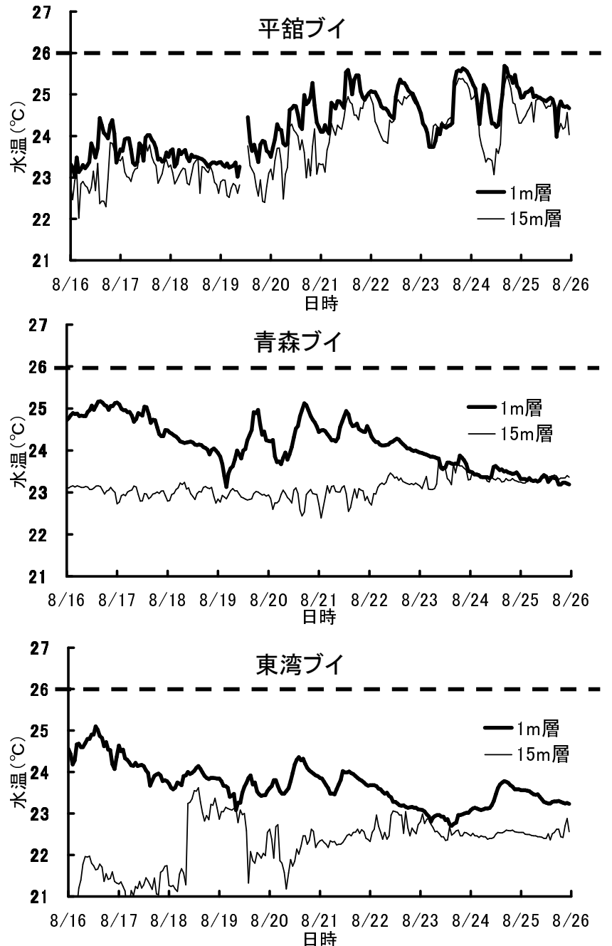
図1 各ブイ1m層、15m層の毎時水温変化
