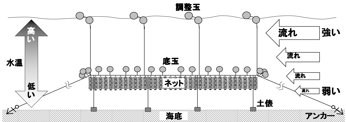
図2 水深による水温や流れの模式図
