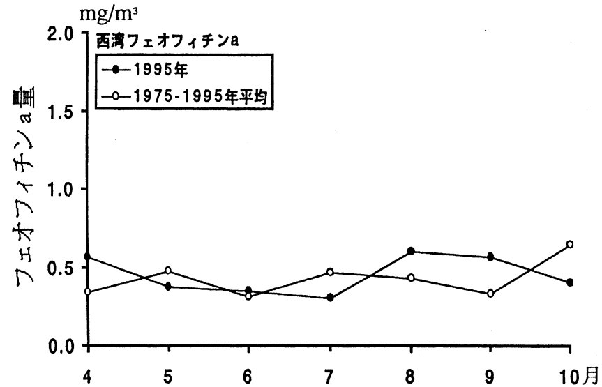
図2 西湾湾央部におけるクロロフィルa、フェオフィチンaの分布状況 (1995年・0、20、40m層平均)
