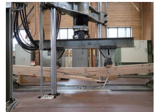
photo: 実大サイズの木材強度試験
