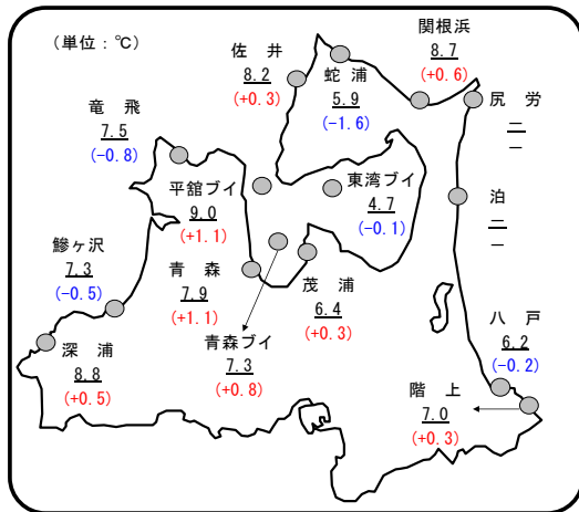
図 定地水温(3月26日~31日) 平均値(平年差)ブイは1m
