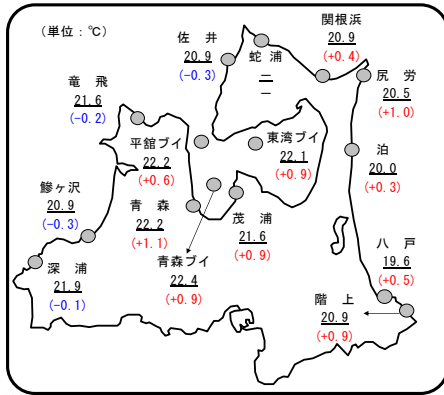
図 定地水温 (9月26日～30日) 平均値 (平年差) ブイは 1 m
