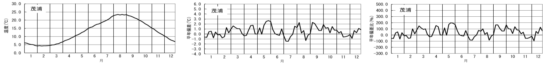
図 5-2. 茂浦定地観測における半月別平均水温、平年偏差及び平年偏差比 (2019 年)
