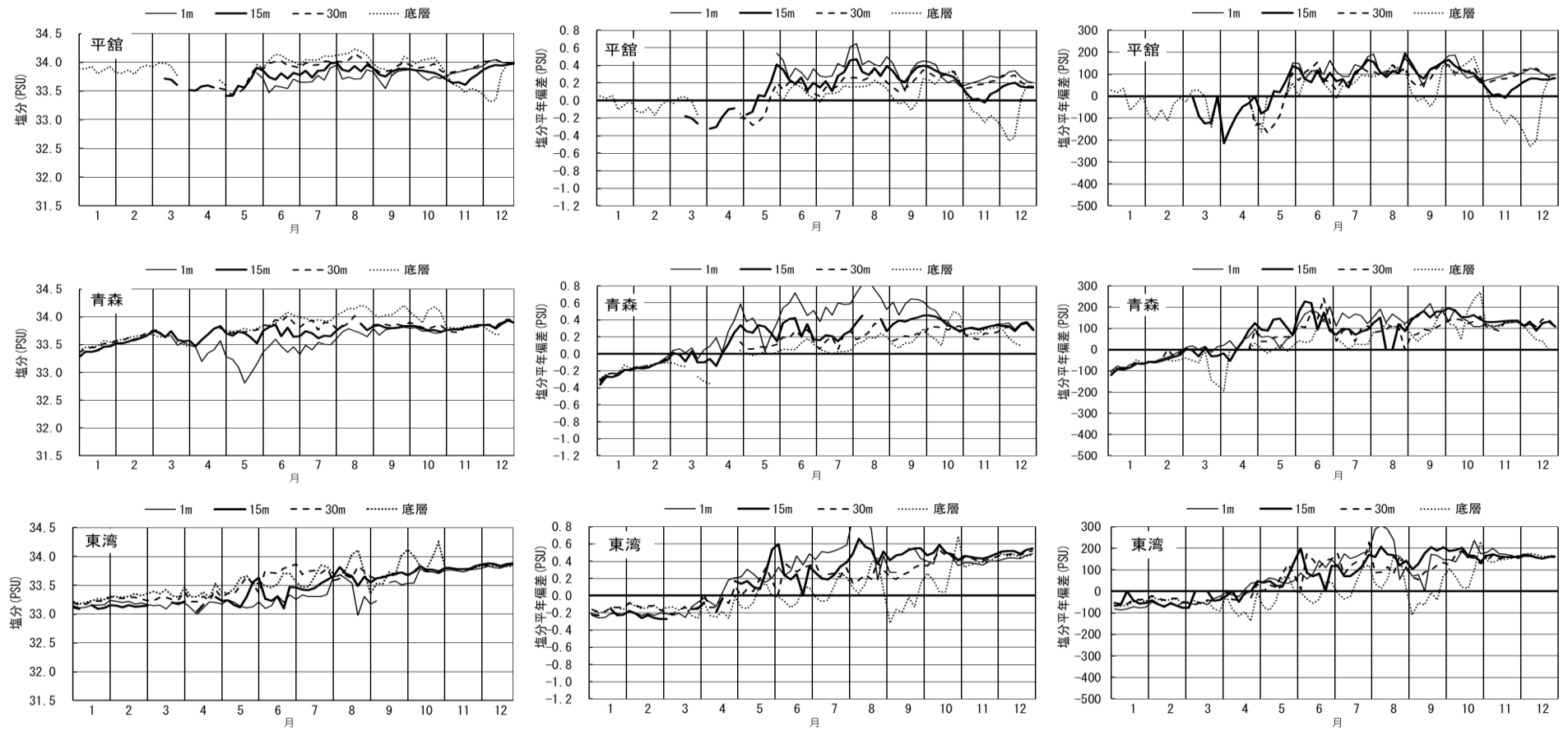
図 6. 各ブイにおける半月別平均塩分、平年偏差及び平年偏差比 (2019 年)
