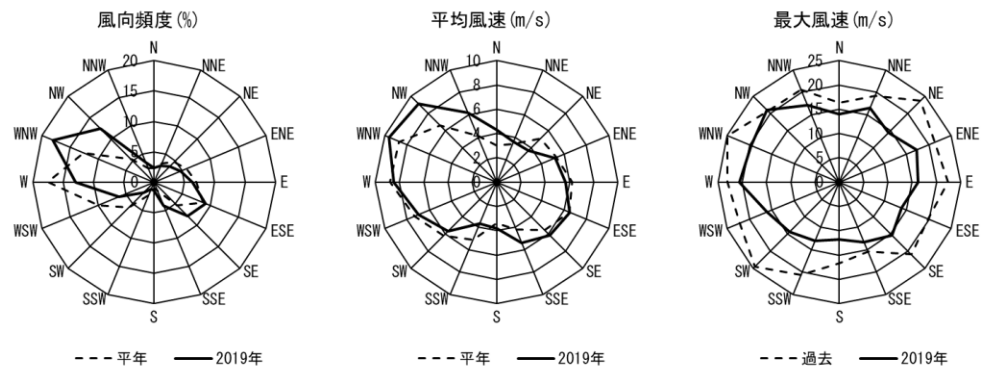
図 3. 東湾ブイ風向別の出現頻度、平均風速及び最大風速 (2019 年)
