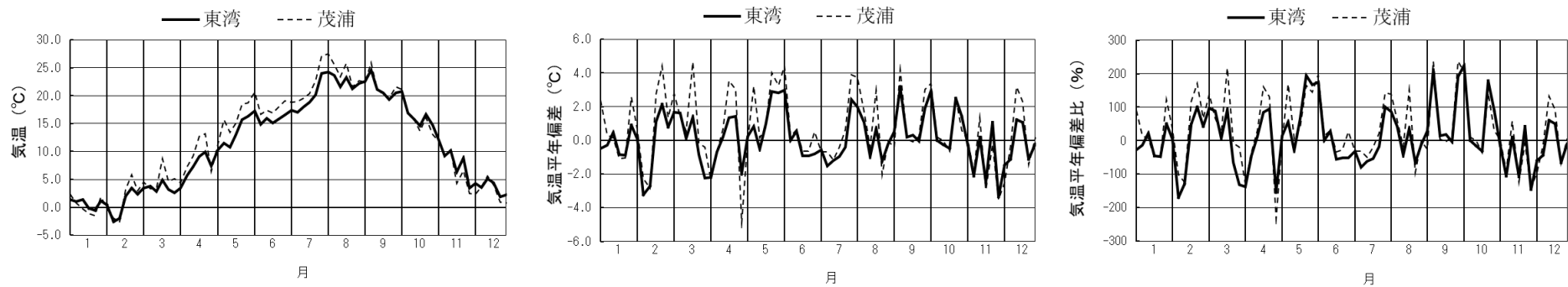
図 2. 東湾ブイと茂浦の半旬別の平均気温、平年偏差及び平年偏差比 (2019 年)
