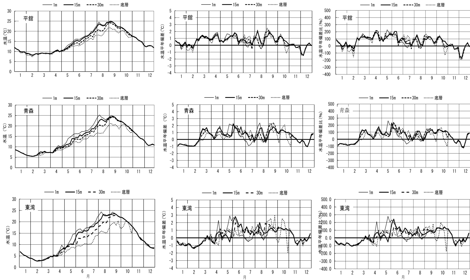
図 5-1. 各ブイにおける半旬別の平均水温、年間偏差及び年間偏差比(2019年)
