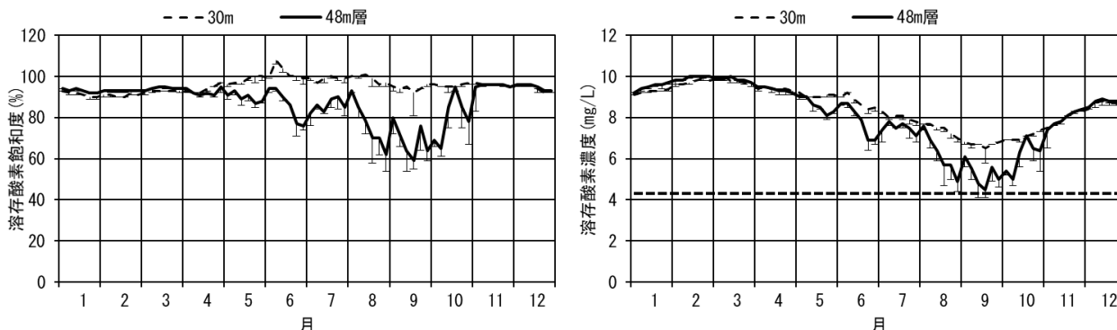
図 7. 東湾ブイ 30m 層及び 48m 層の半旬別溶存酸素の推移(左:飽和度 右:濃度) (2019 年)
