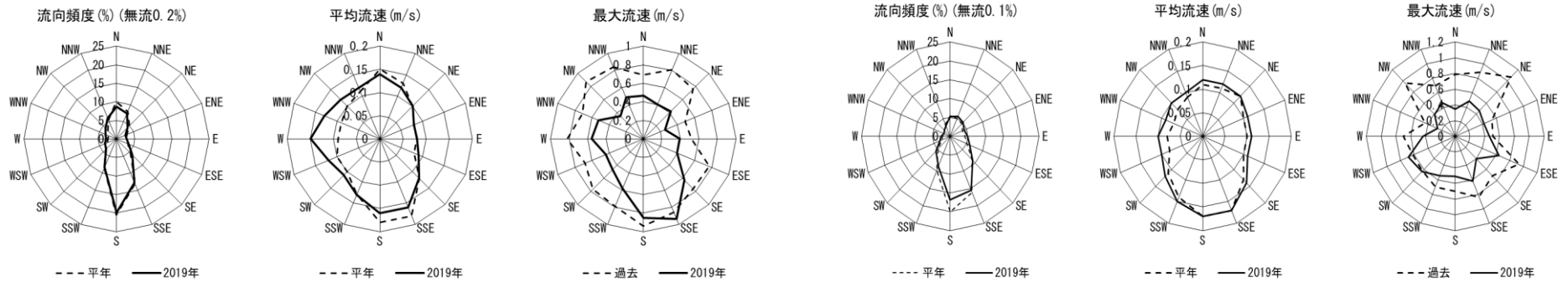
図 8. 平館ブイ流向別出現頻度、平均流速及び最大流速(左:15m層 右:40m層) (2019年)
