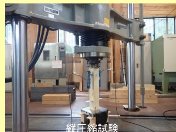
縦圧縮試験
