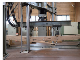
photo: 実大サイズの木材強度試験
