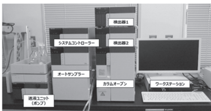
導入装置：高速液体クロマトグラフ （Prominence GPC システム，SHIMADZU）
