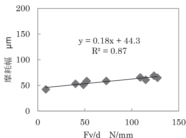
S45Cの工具寿命予測線図
