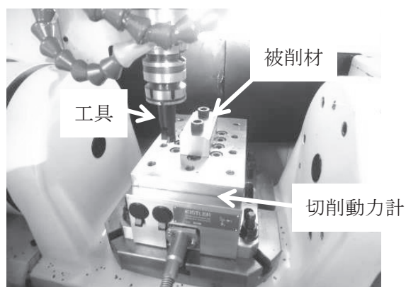
実験装置
