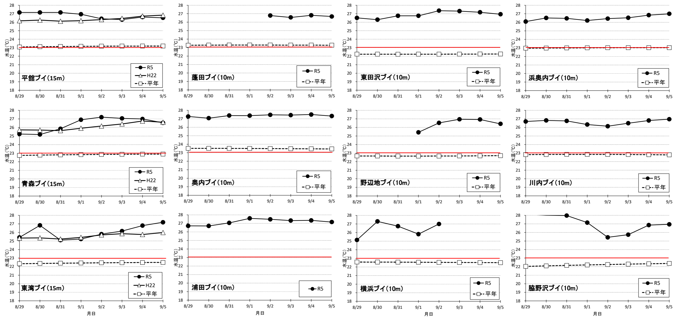
図4 海況自動観測ブイ・水温観測ブイでの中層(10~15m層)の日平均水温 ※平館、青森、東湾ブイは平成22年の水温も掲載
