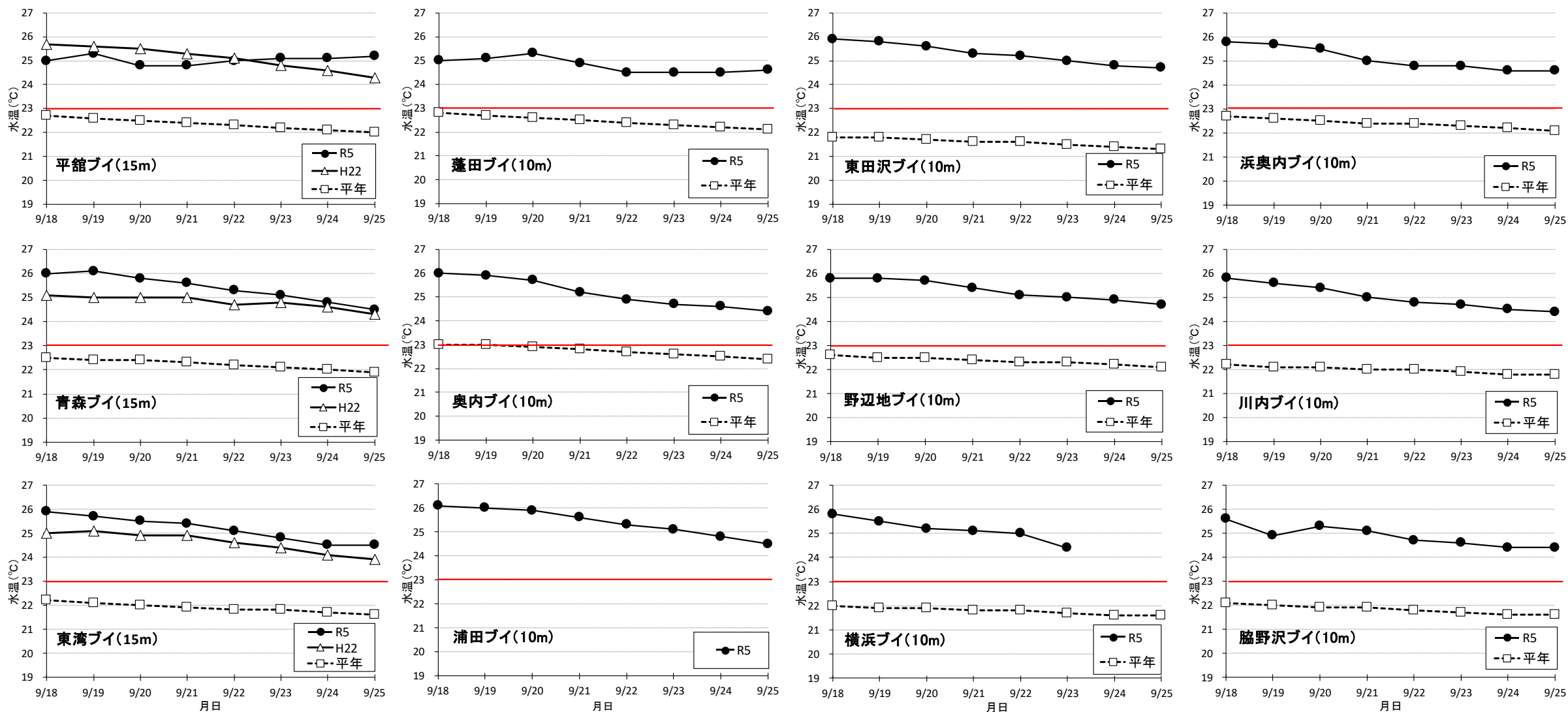
図4 海況自動観測ブイ・水温観測ブイでの中層(10~15m層)の日平均水温
