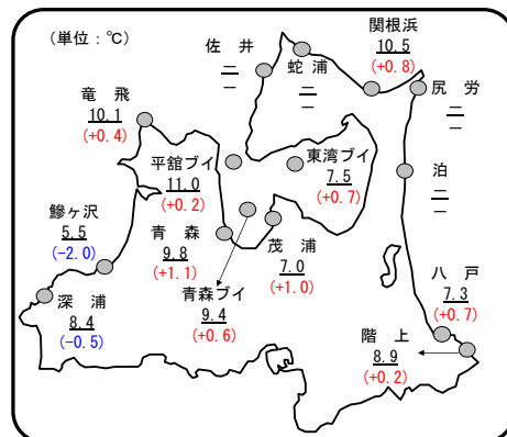
図 定地水温(1月6日～10日) 平均値(平年差)ブイは1m
