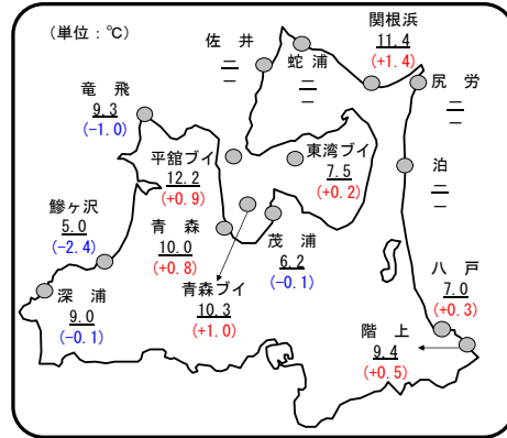
図 定地水温(1月1日～5日) 平均値(平年差)ブイは1m
