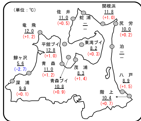
図 定地水温(12月26日～31日) 平均値(前年差)ブイは1m
