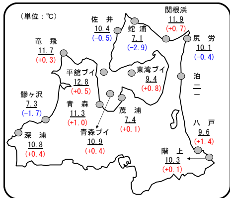
図 定地水温(12月21日～25日) 平均値(前年差)ブイは1m
