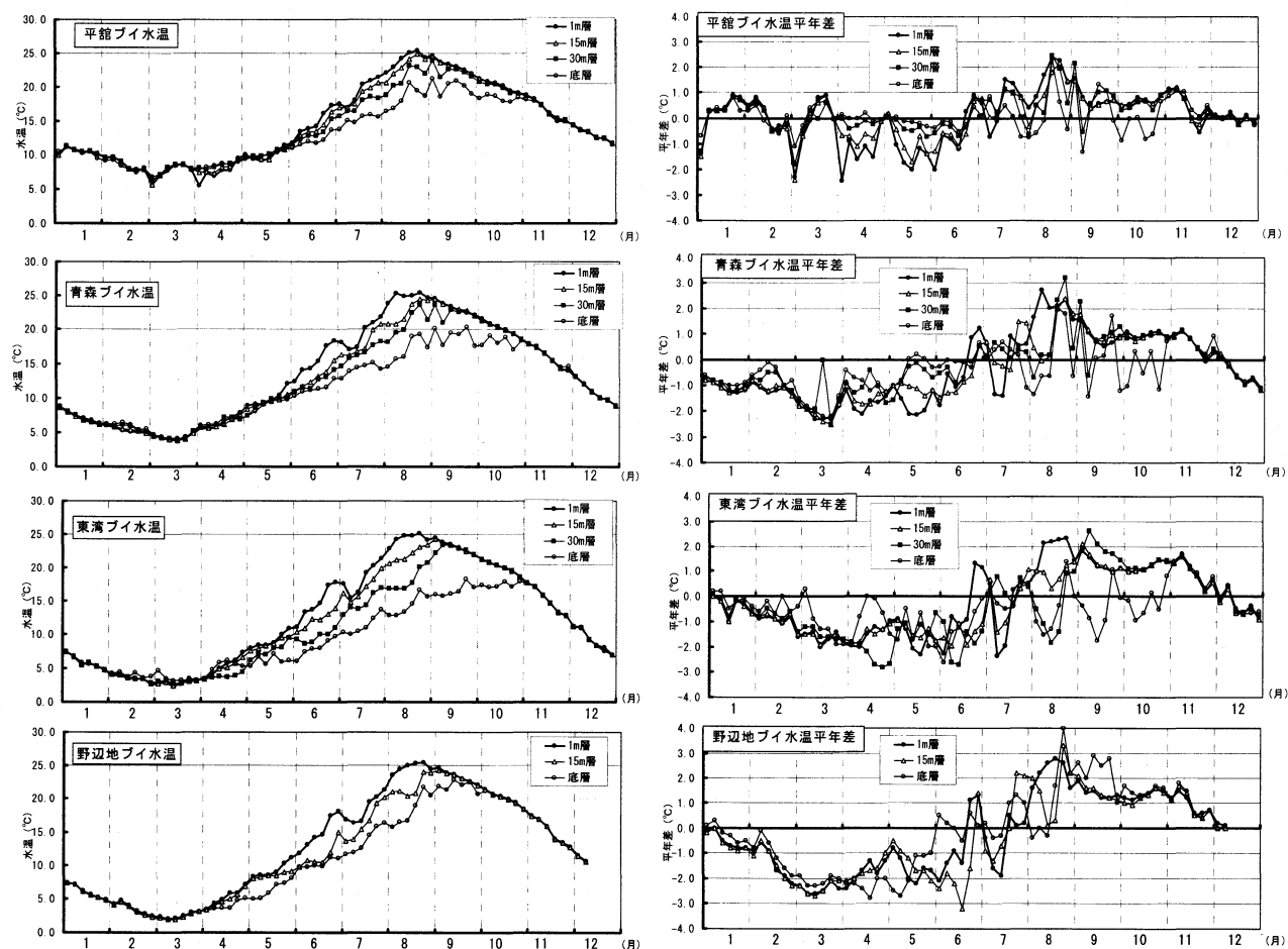
図2 ブイ別全層の半月別平均水温とその平年差
