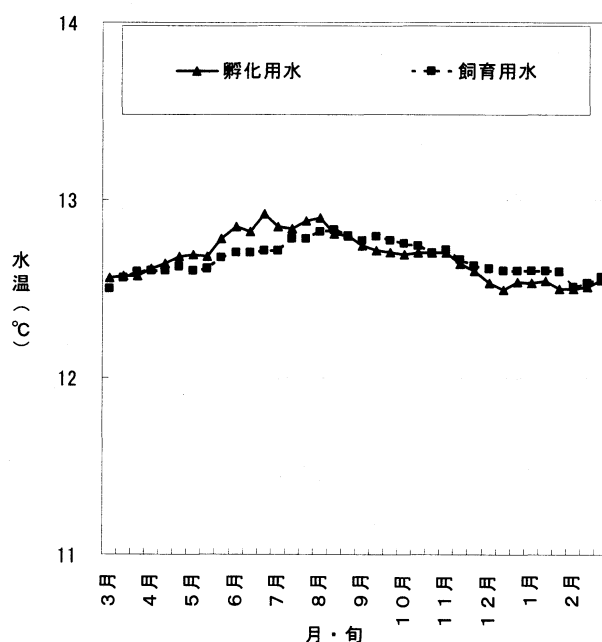
図 3 旬別水温の推移
