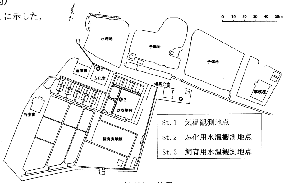
図 1 観測点の位置
