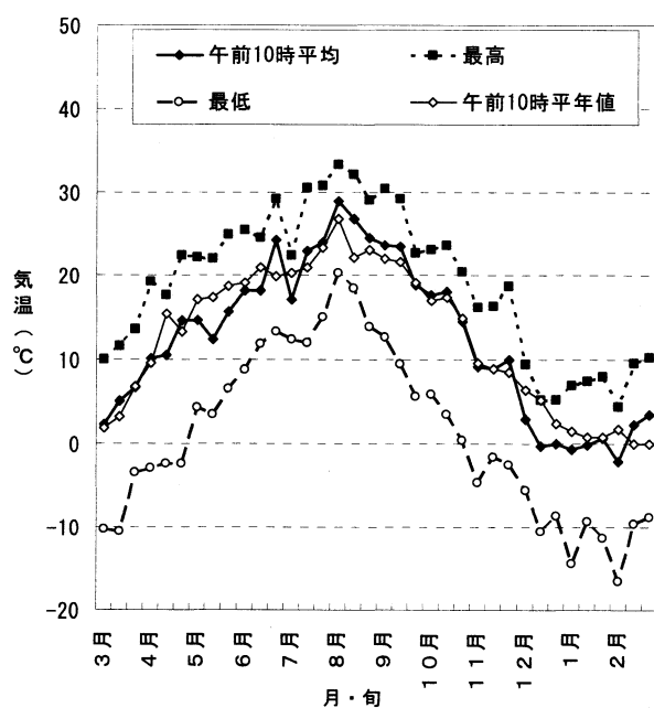
図 2 旬別気温の推移
