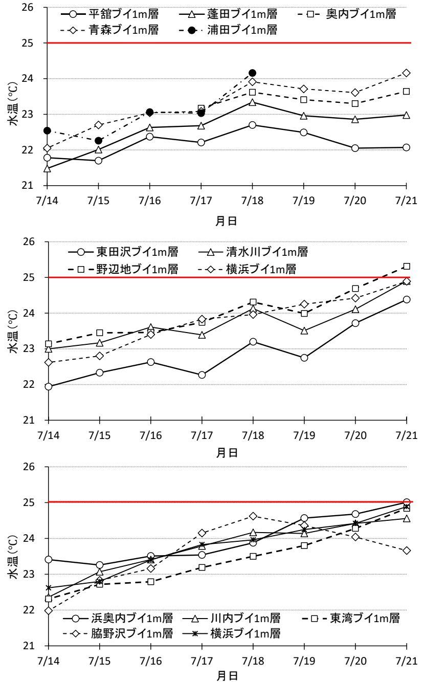
図1 1m層の海況自動観測ブイと水温観測ブイの日平均水温の変化
