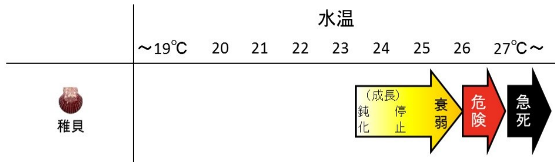
図2 ホタテガイ稚貝の成長と生残率に与える水温の影響
