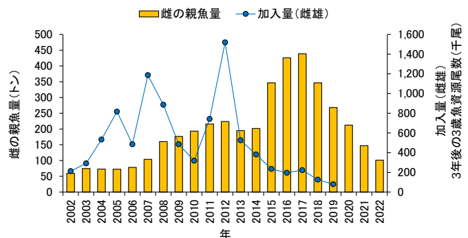
図 6. 青森県日本海側におけるムシガレイの雌親魚量と加入量の経年変化
