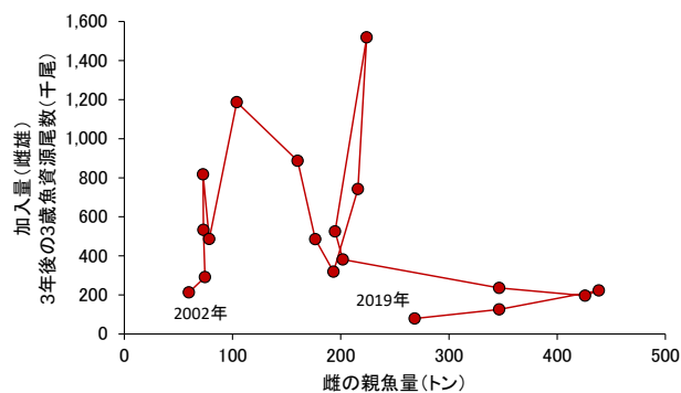
図 7. 青森県日本海側におけるムシガレイの雌親魚量と加入量との関係
