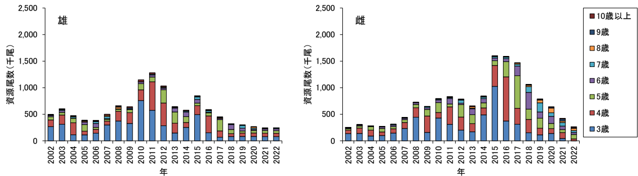
図 4. 青森県日本海側におけるムシガレイの年齢別資源尾数の推移（左図：雄、右図：雌）
