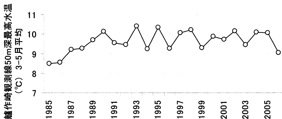
図 4 青森県日本海側舮作崎西方沖の定線観測による 50m 深最高水温の 3～5 月平均値
