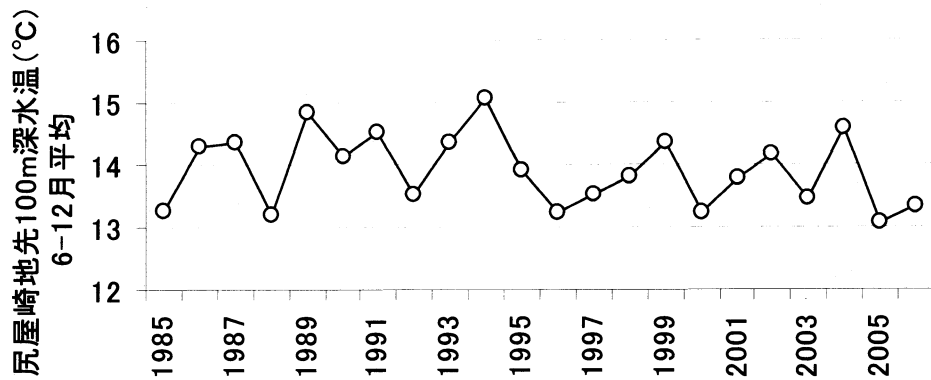
図 6 青森県尻屋崎東方沖合 12km の定線観測地点 (SY1) における 100m 深水温の 6~12 月平均値
