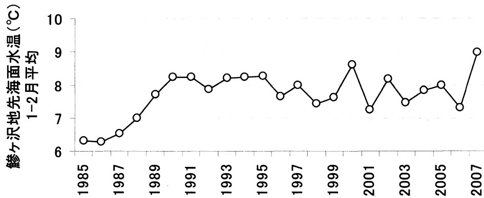
図 7 青森県日本海側鯺ヶ沢地先における海面水温の 1~2 月平均値
