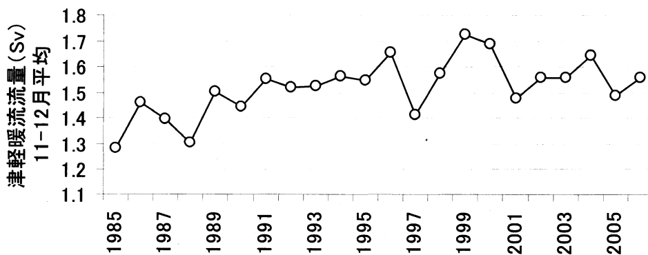
図 9 津軽暖流流量 (深浦と函館の水位差より推定) の 11~12 月平均値
