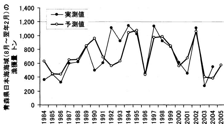
図 16 津軽暖流の流量から予測した青森県日本海海域の実測値と予測値
