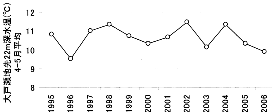
図 5 青森県日本海側深浦町大戸瀬地先水深 25m 地点における海底上 3m 水温の 4～5 月平均値
