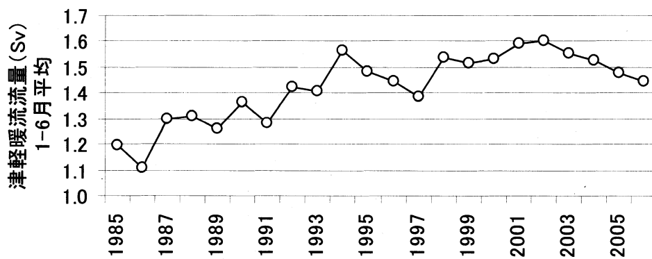
図 8 津軽暖流流量 (深浦と函館の水位差より推定) の 1~6 月平均値
