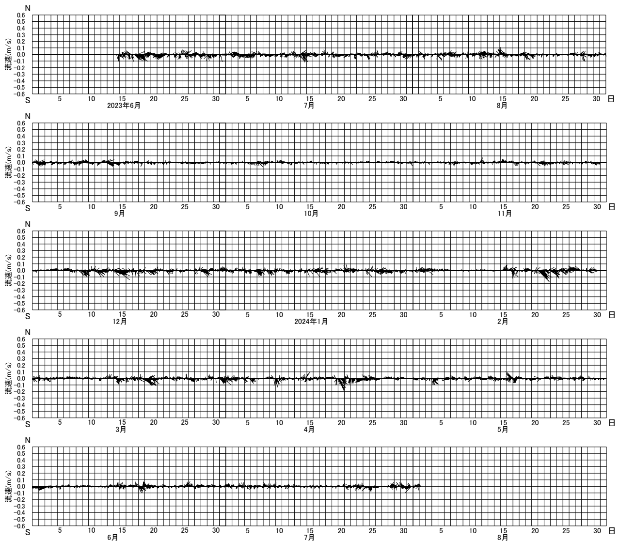
図 30. 試験期間中の流向流速の推移(野辺地)
