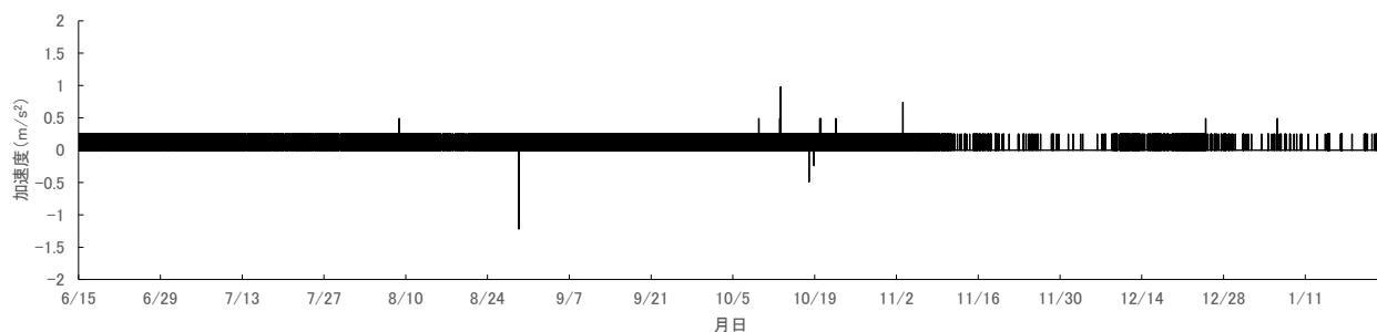
図 40. 試験期間中の鉛直方向の加速度の推移 (川内)
