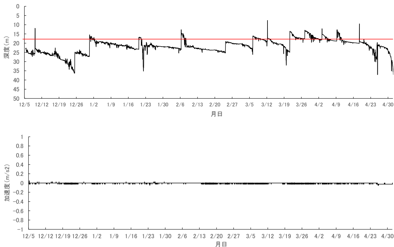
図 8. 茂浦晩期の深度及び鉛直方向の加速度の推移（赤線は設定した幹綱深度）
