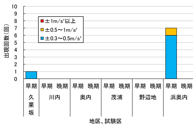
図 13. 試験期間中における幹綱鉛直方向の加速度の値別出現回数
