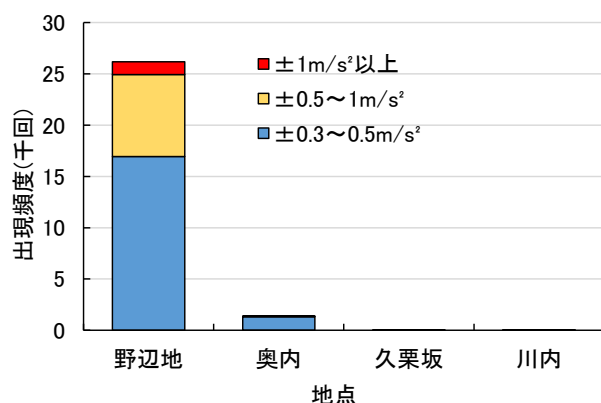
図 32. 各地点の幹綱鉛直方向の加速度 \pm 0.3 \text{ m/s}^2 以上の絶対値の出現頻度
