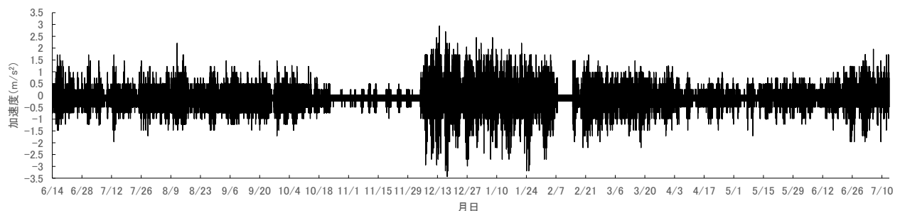
図 31. 試験期間中の鉛直方向の加速度の推移(野辺地)
