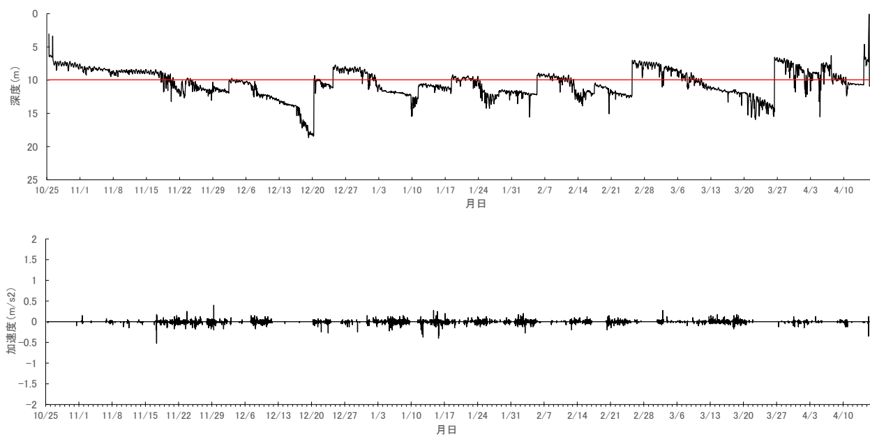
図 11. 浜奥内早期の深度及び鉛直方向の加速度の推移 (赤線は設定した幹綱深度)
