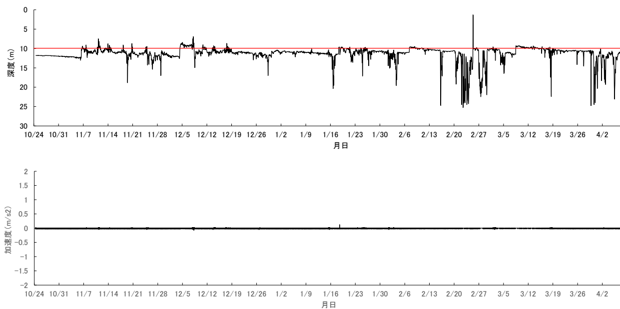
図 9. 野辺地早期の深度及び鉛直方向の加速度の推移 (赤線は設定した幹綱深度)
