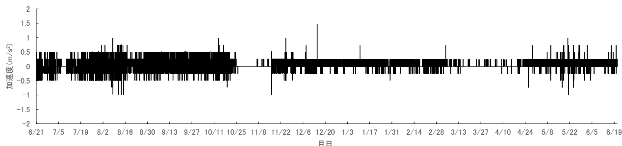
図5. 試験期間中の鉛直方向の加速度の推移(奥内)
