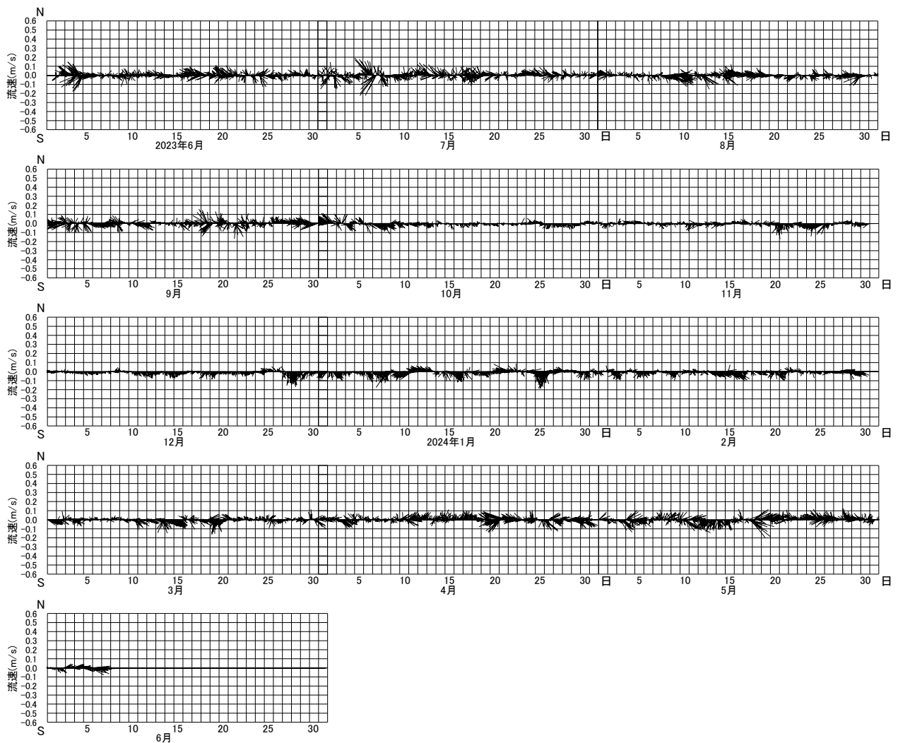
図 39. 試験期間中の流向流速の推移(川内)
