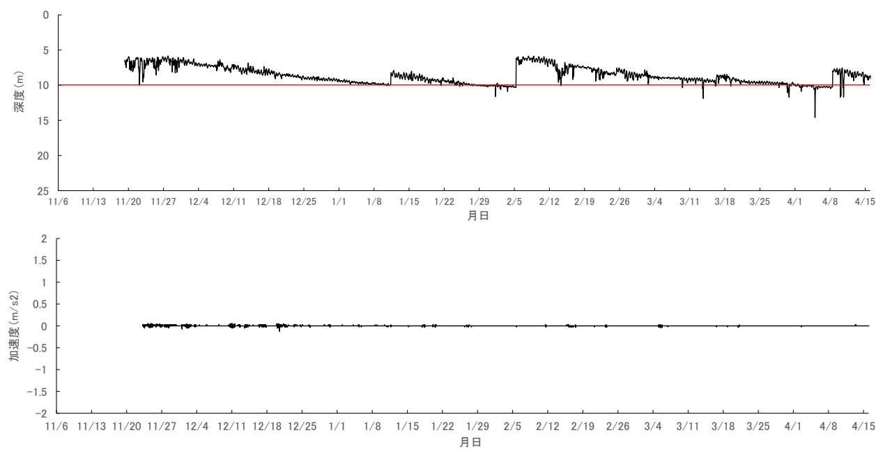
図 12. 浜奥内晩期の深度及び鉛直方向の加速度の推移 (赤線は設定した幹綱深度)
