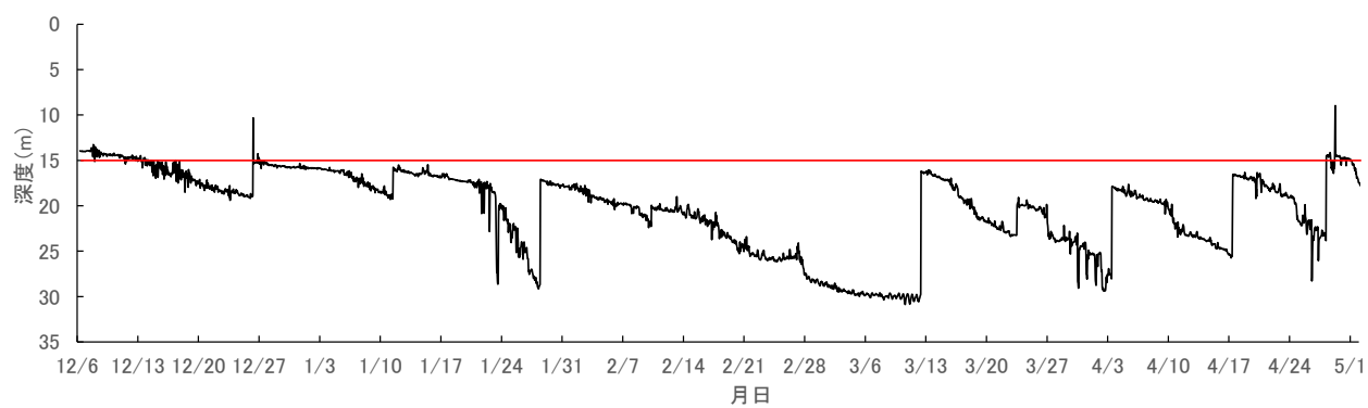
図 5. 奥内早期の深度及び鉛直方向の加速度の推移 (赤線は設定した幹綱深度)
