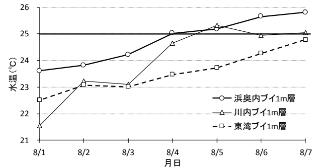
図1 1m層の海況自動観測ブイと水温観測ブイでの日平均水温の変化
