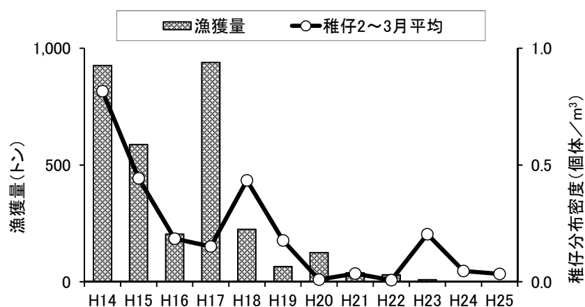
図2 2～3月のイカナゴ平均稚仔分布密度（調査地点③④⑧⑨の平均値）と漁獲量（三厩～佐井村漁協）の経年変化
