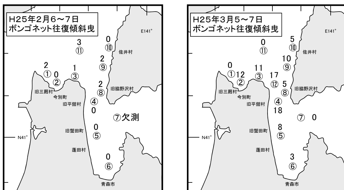
図1 ボンゴネット水深0～50m 往復傾斜曳によるイカナゴ稚仔の1網当りの採集個体数（①～⑫：調査地点 数字：採集個体数）
