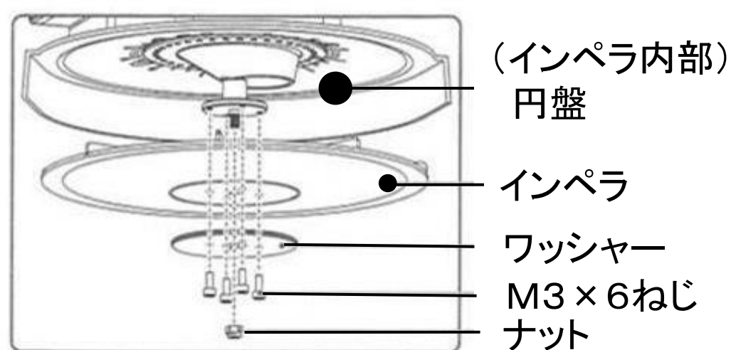
図3-5 粒剤散布機の内部構造 (DJI社 MG粒剤散布機ユーザーガイドより)
