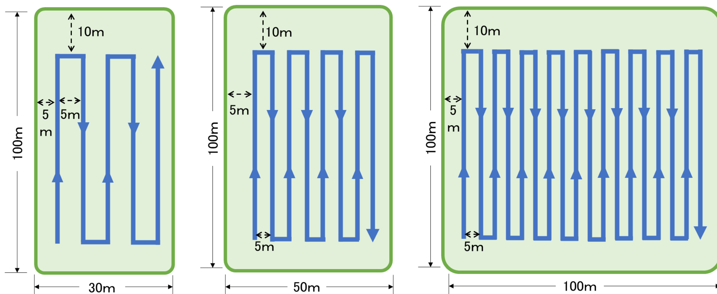
図3-8 「豆つぶ剤」散布における円盤目盛3での散布経路の例
