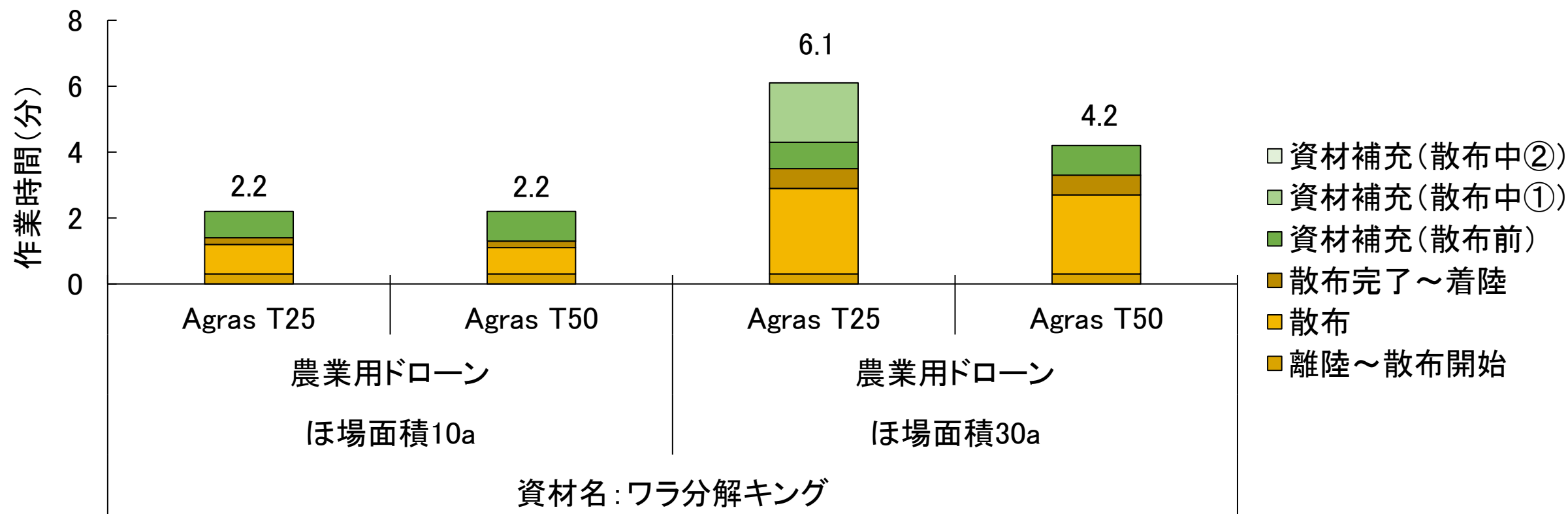
図3-30 農業用ドローンによる稲わら分解資材の散布に係る作業時間
