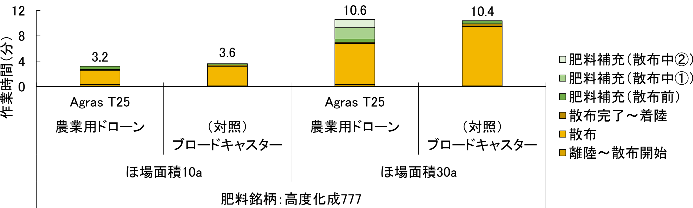
図4-2 農業用ドローンによる大豆作の基肥散布に係る作業時間
