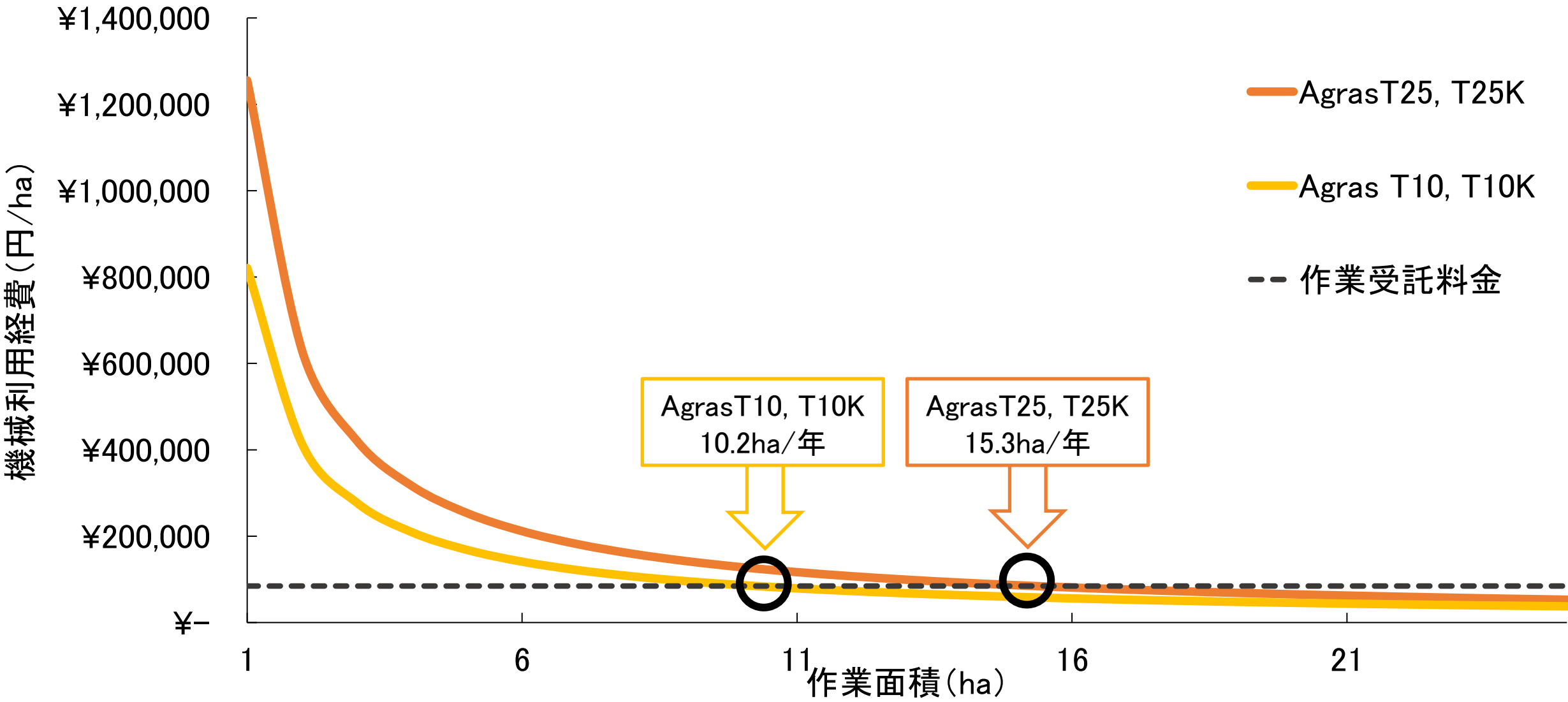
図5-1 利用面積と機械利用経費の関係性
