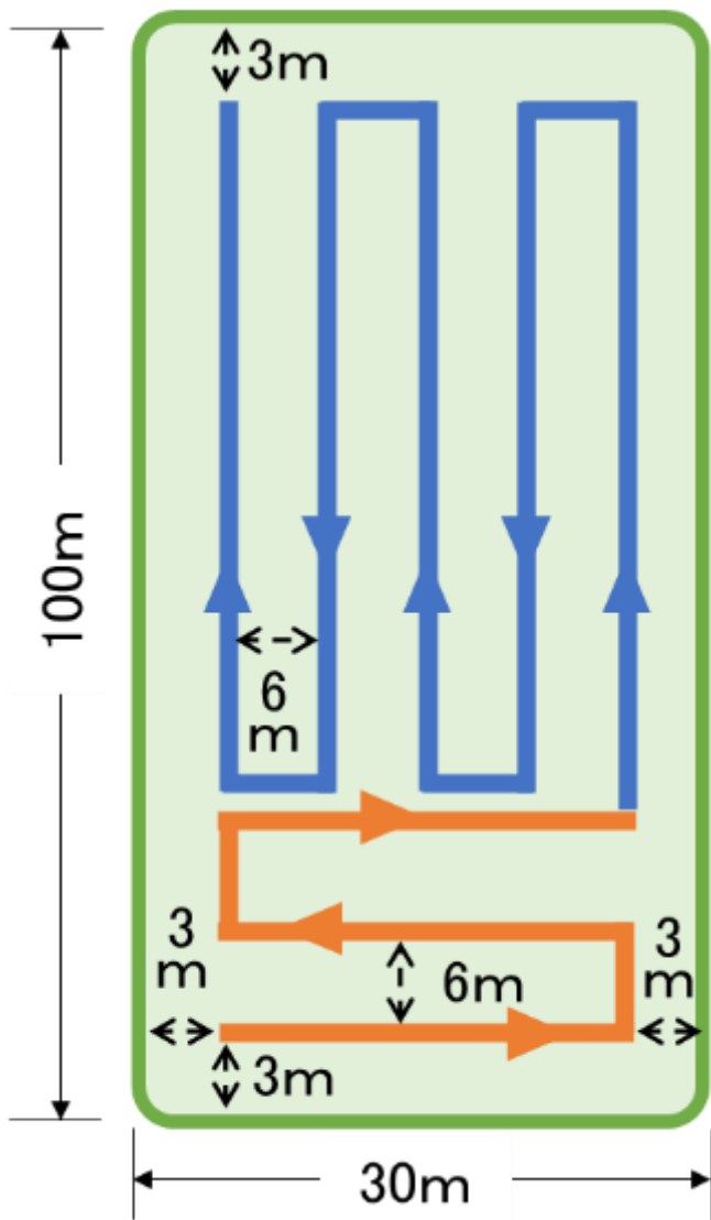
図3-23 散布幅6.0mでの散布経路の例
