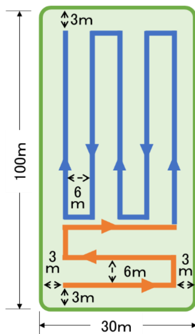
図4-1 散布幅6.0mでの散布経路の例
