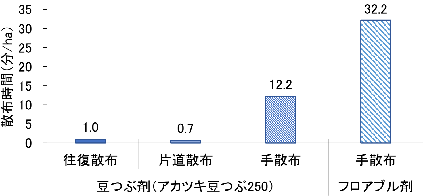
図3-17 農業用ドローンによる「豆つぶ剤」の散布時間
