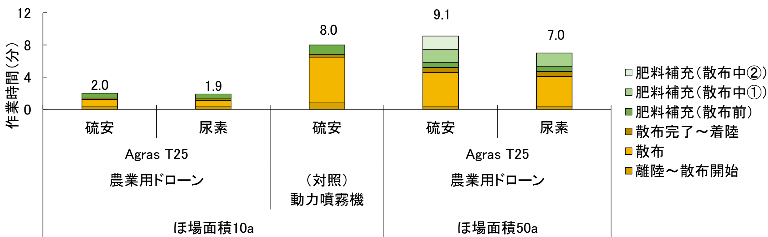
図3-24 農業用ドローンによる水稻作の追肥に係る作業時間
