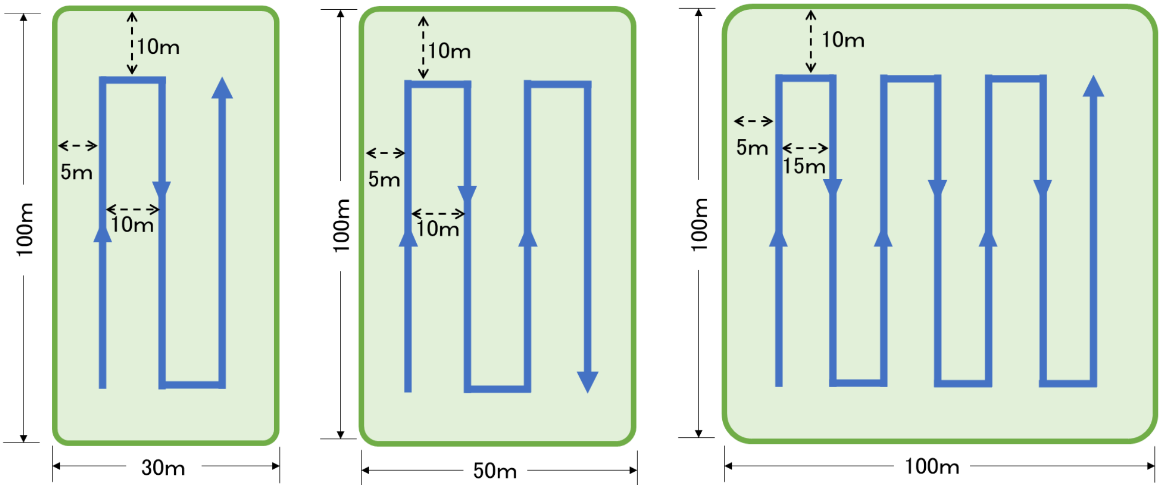
図3-7 「豆つぶ剤」散布における円盤目盛15での散布経路の例
