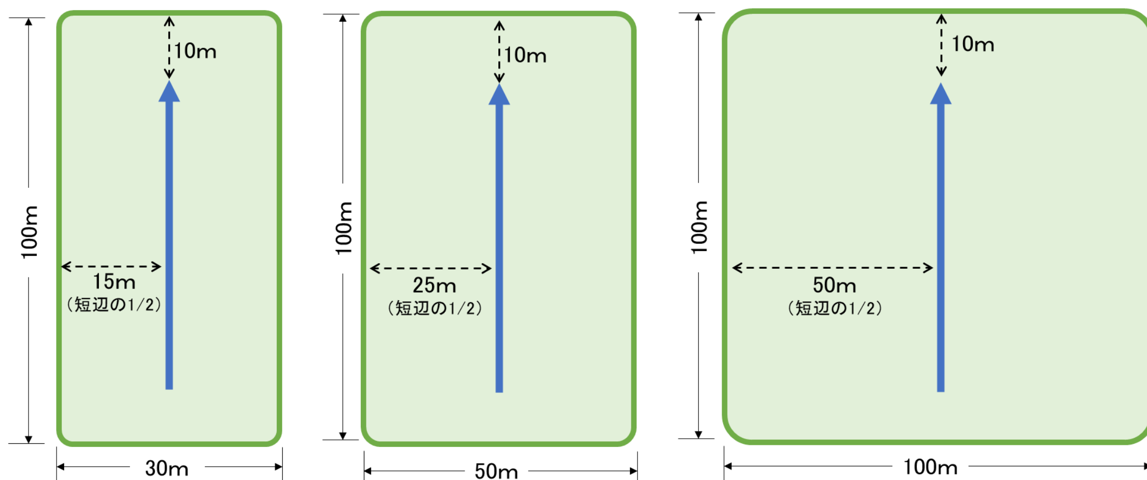
図3-15 「豆つぶ剤」散布における片道散布での散布経路の例
