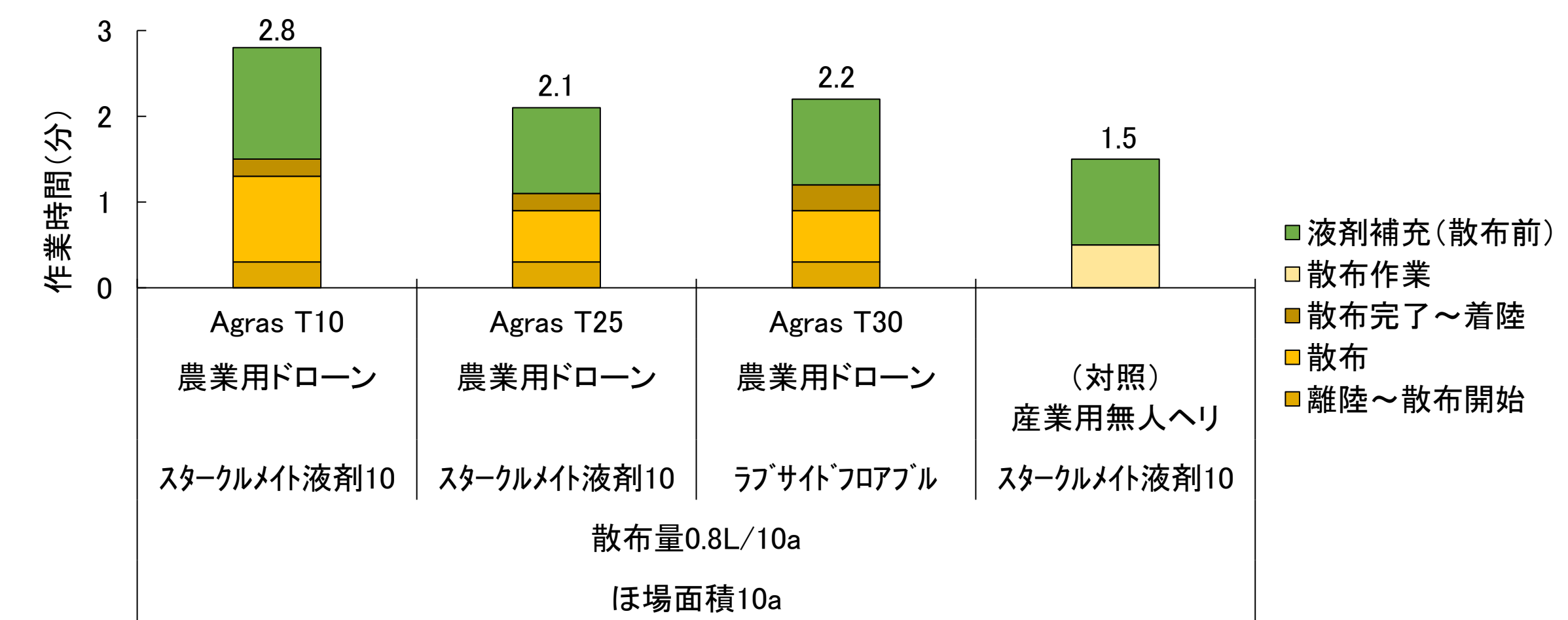
図3-27 農業用ドローンによる水稲作の液剤散布に係る作業時間
