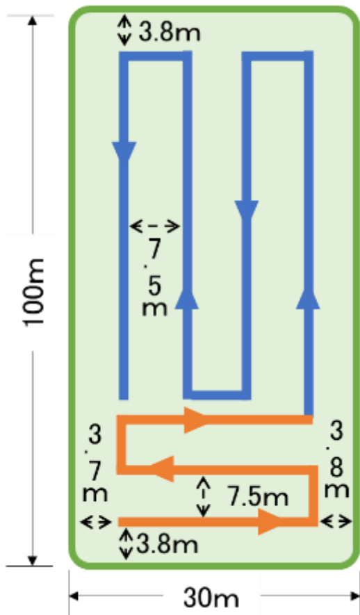
図4-4 散布幅7.5mでの散布経路の例
