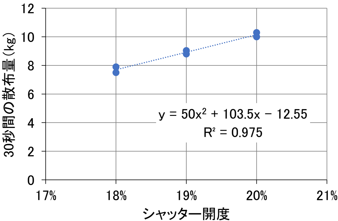
図3-29 AgrasT25, T50における稲わら分解資材(ワラ分解キング)とシャッター開度の関係
