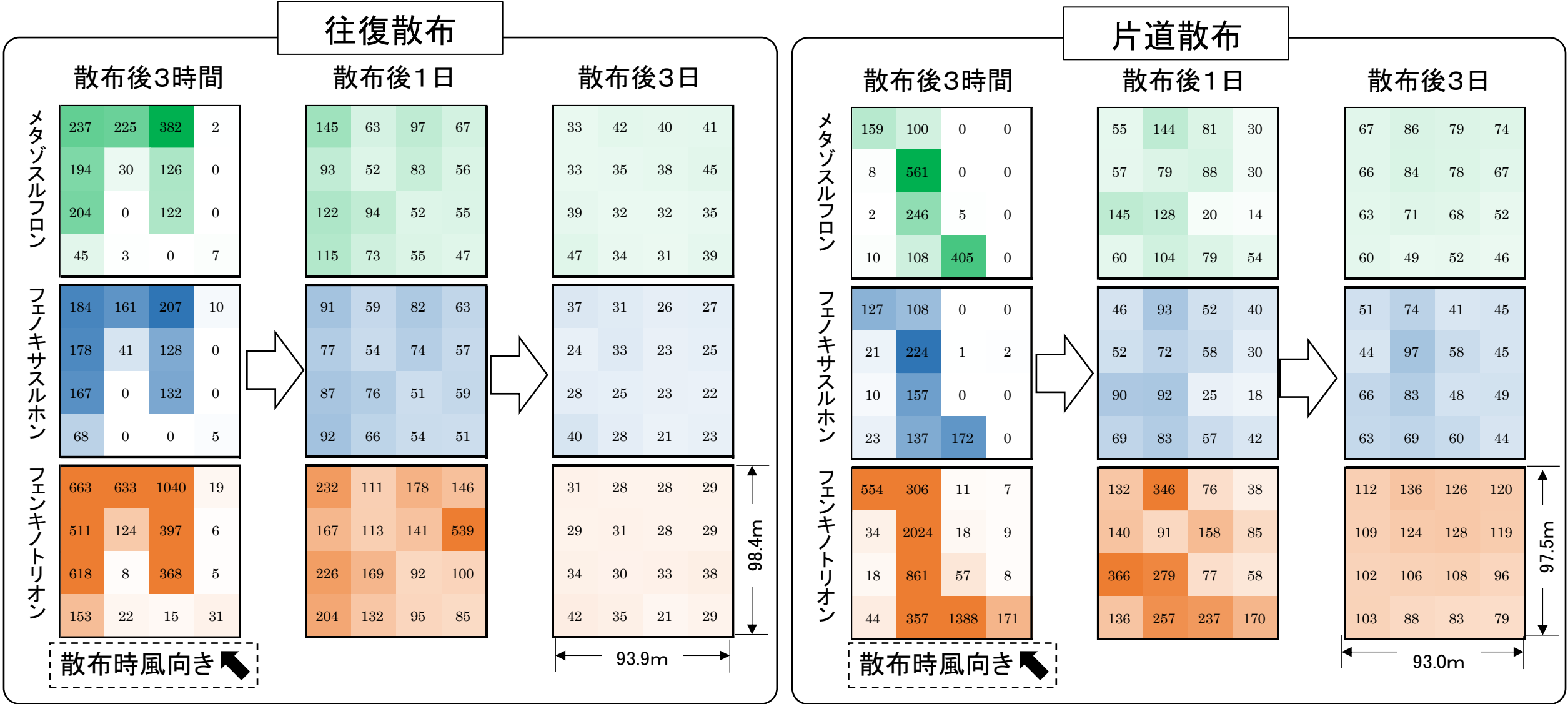
図3-19 往復散布と片道散布における有効成分の拡散性 注 図中の数字は各成分の田面水中の濃度(ppb)を示す。
