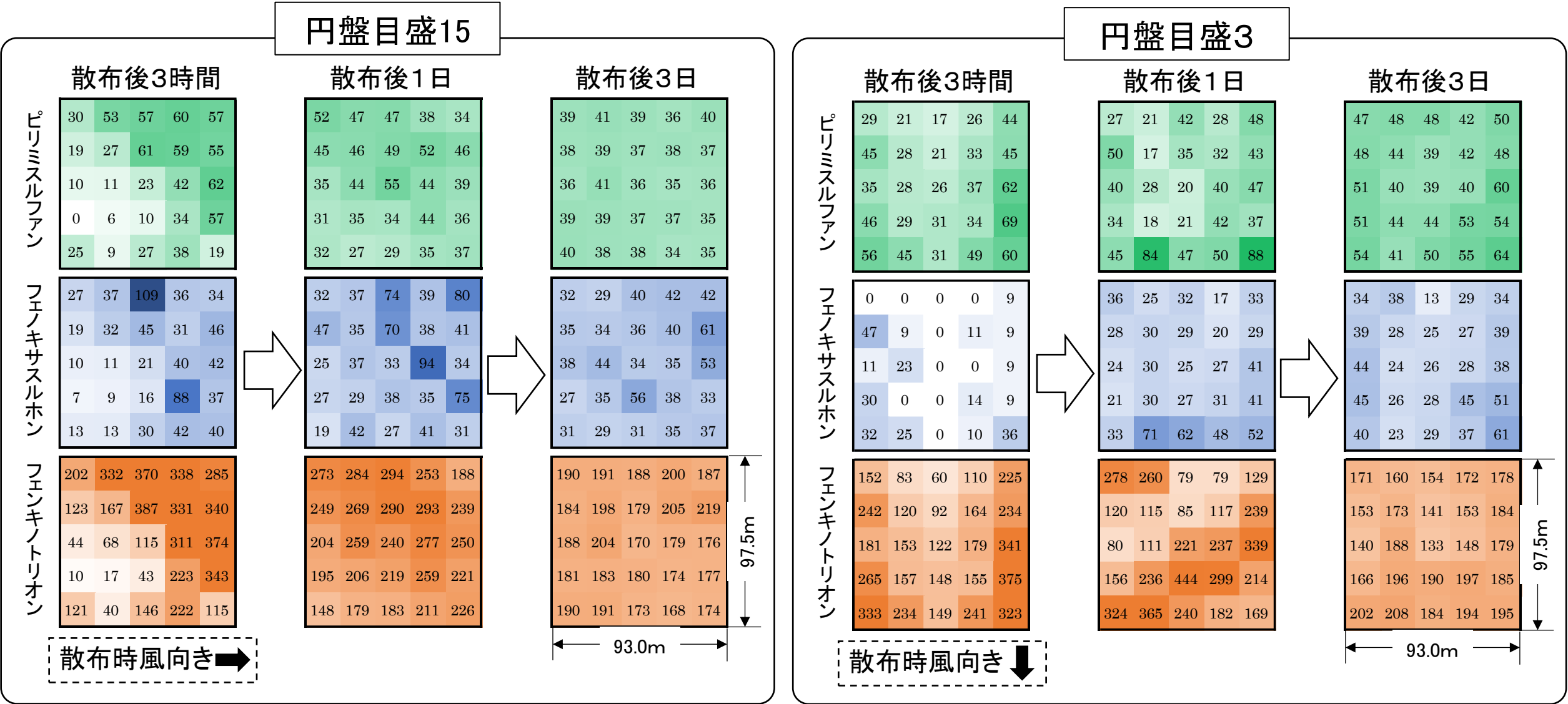
図3-12 円盤目盛15と円盤目盛3における有効成分の拡散性 注 図中の数字は各成分の田面水中の濃度(ppb)を示す
