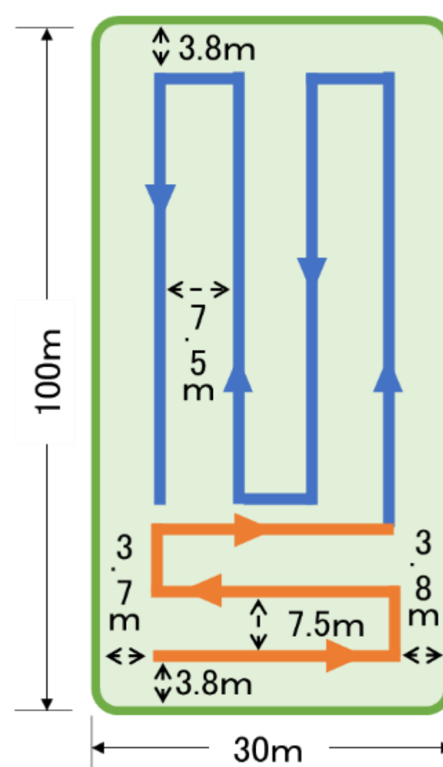
図3-26 散布幅7.5mでの散布経路の例
