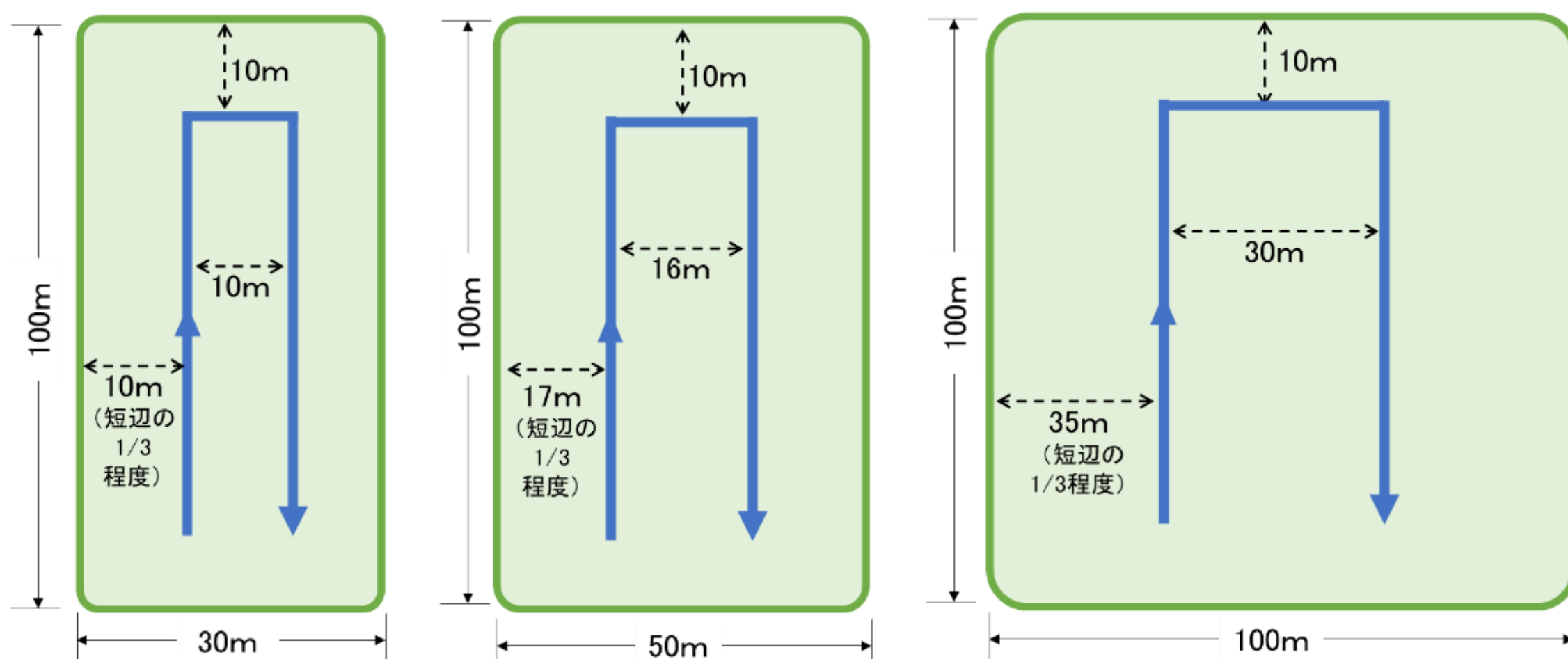
図3-14 「豆つぶ剤」散布における往復散布での散布経路の例
