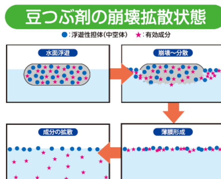
図3-2 「豆つぶ剤」の成分の拡散の仕組み
