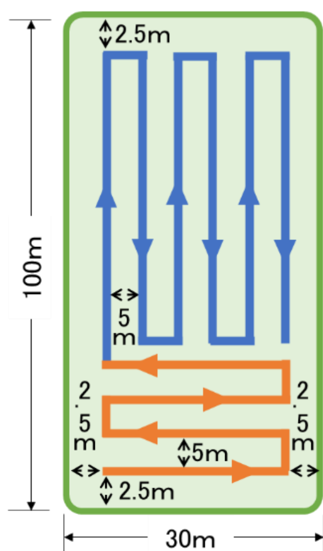
図3-25 散布幅5.0mでの散布経路の例
