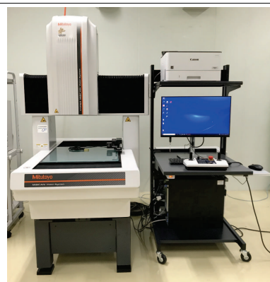
装置外観
